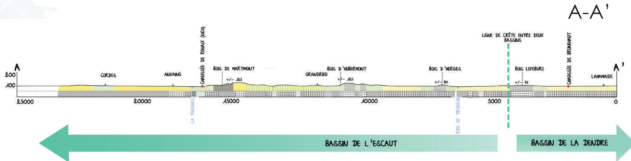
Fig. 29 : Coupe AA' schématique occupation du sol, type de sol et relief ( Source : DR(EA) 2 M; sur base des données de l'IGN )
